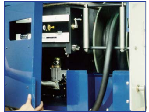
後部機械室に全ての機材をコンパクトに 収納
