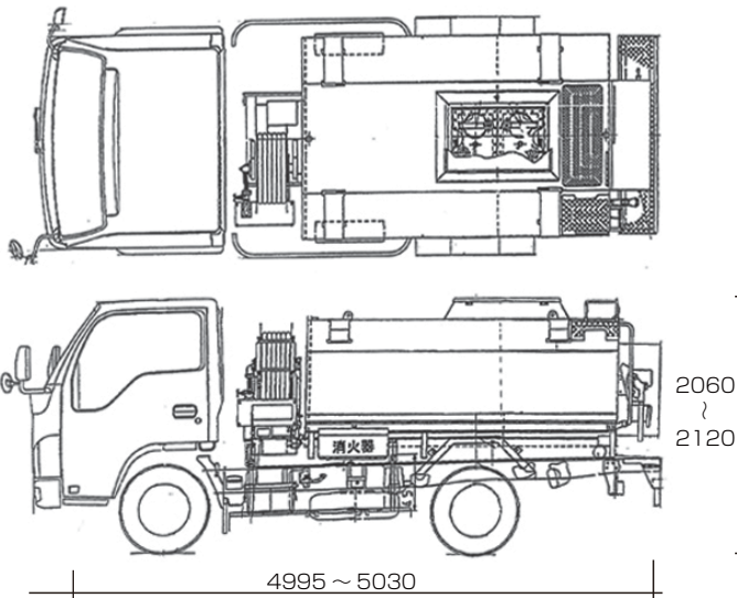
外観寸法図
